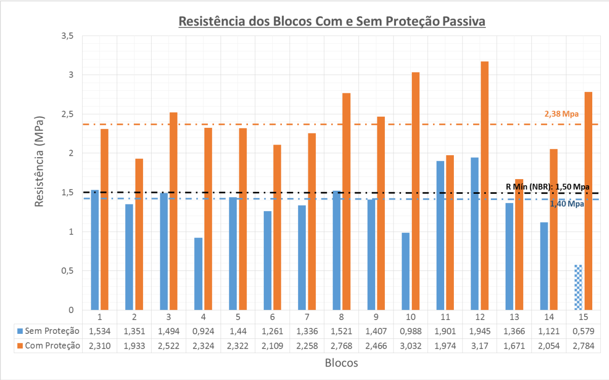
Figura 42 – Comparativo das resistências à compressão para os blocos com e sem proteção passiva, tipos 3 e 4 respectivamente.
