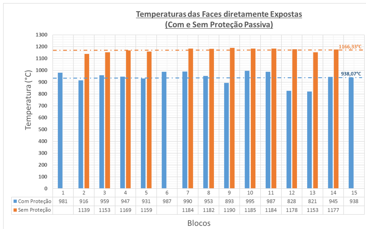
Figura 39 – Comparativo das temperaturas das faces diretamente expostas para os blocos com e sem proteção passiva, tipos 3 e 4 respectivamente.
